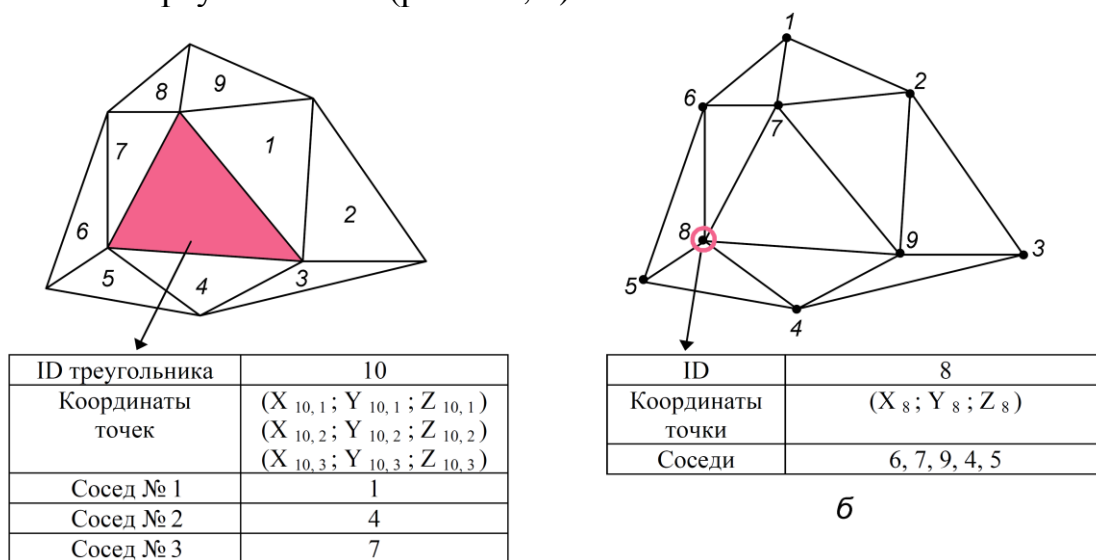
Рис. 2.8. Способы хранения TIN-модели по треугольникам (а): 1 – 9 – треугольники, определяющие TIN-модель, и по точкам (б): 1 – 9 – точки (узлы) TIN-модели
