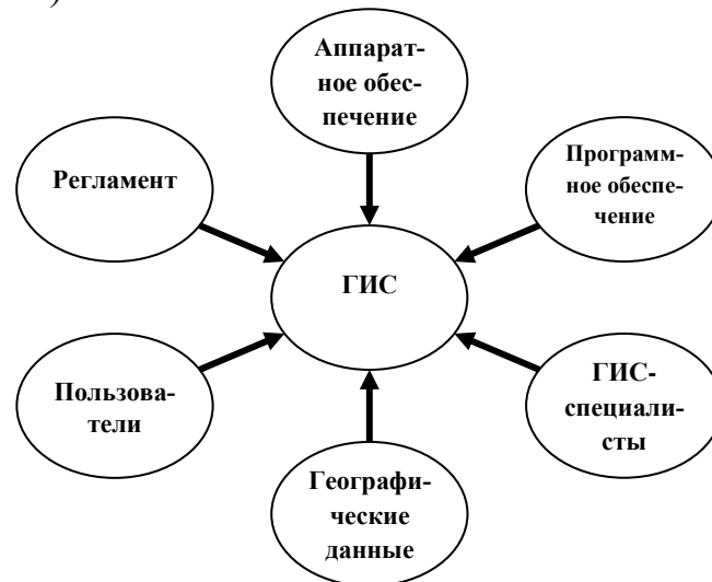
Рис. 1.1. Компоненты ГИС
